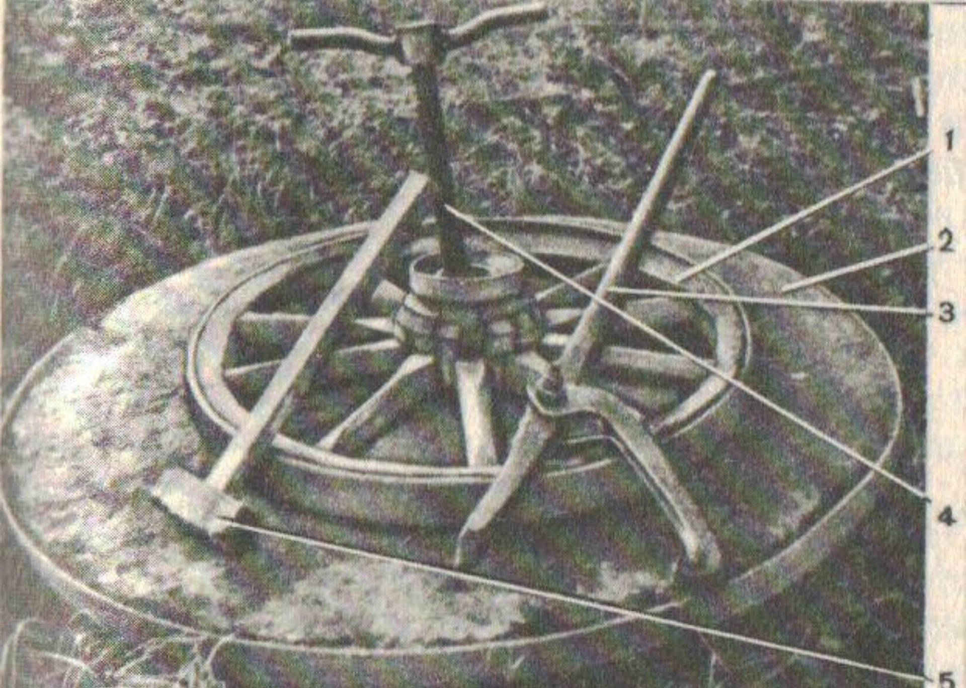
«Камень» для ошиновки колес
