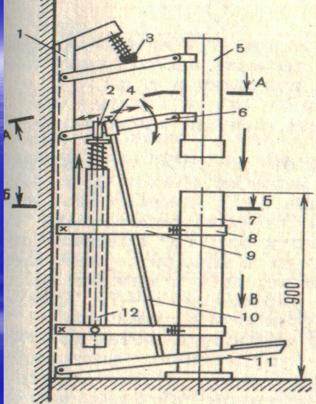
Молот с ножным приводом
