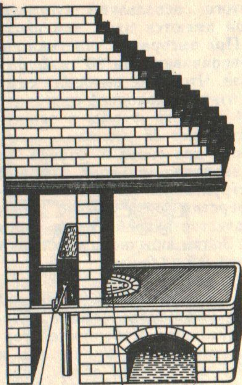
Горн с кирпичным зонтом
