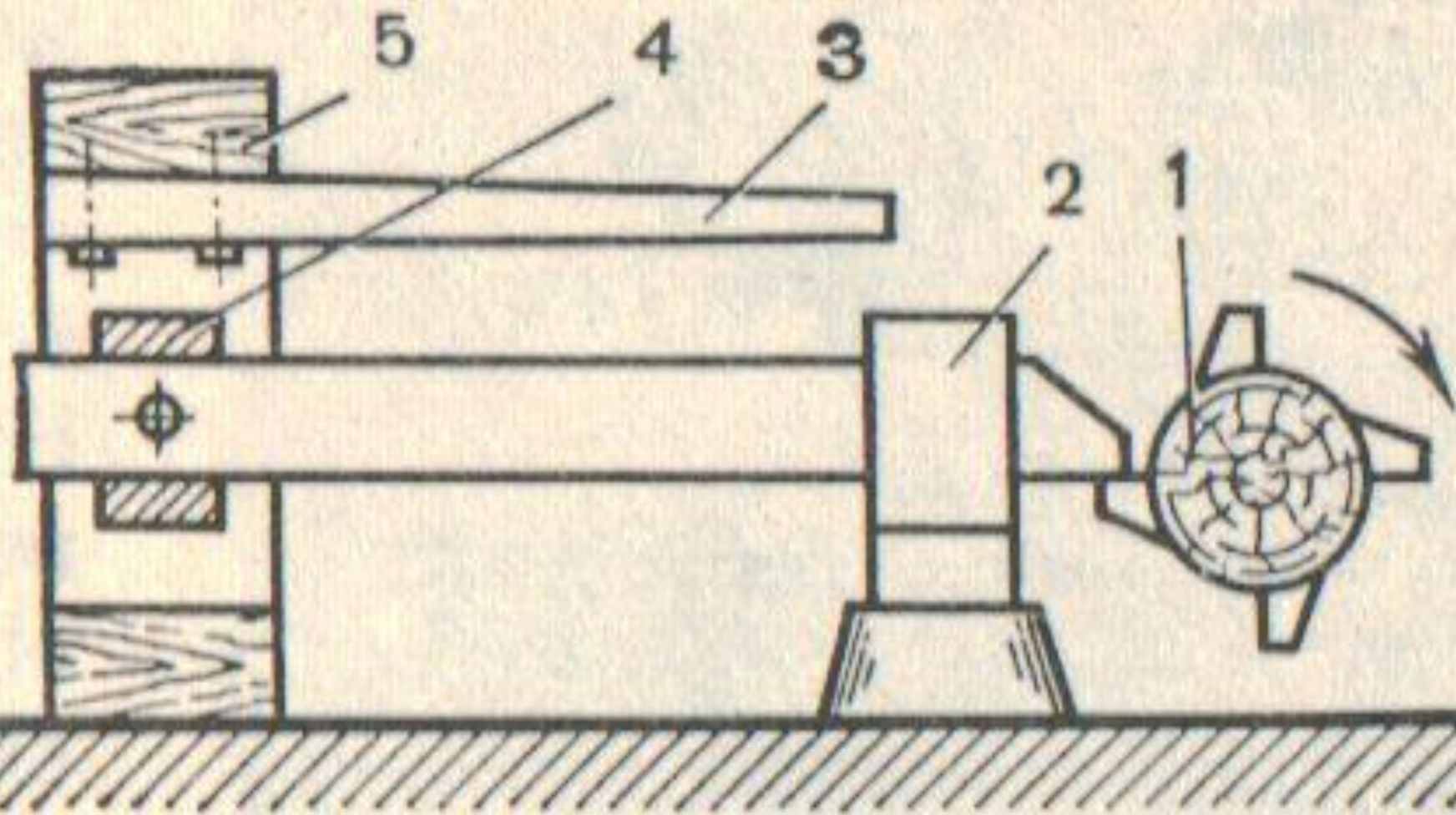
Лобовой молот
